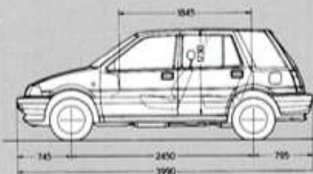
Civic 1,5 L Shuttle
