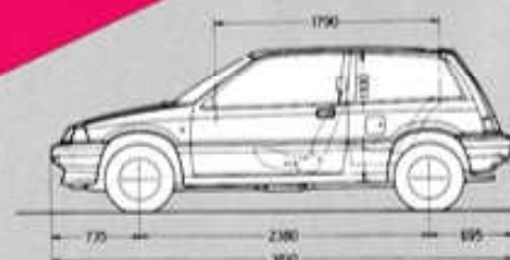
Civic 1,3 L et 1,5 L "S"
