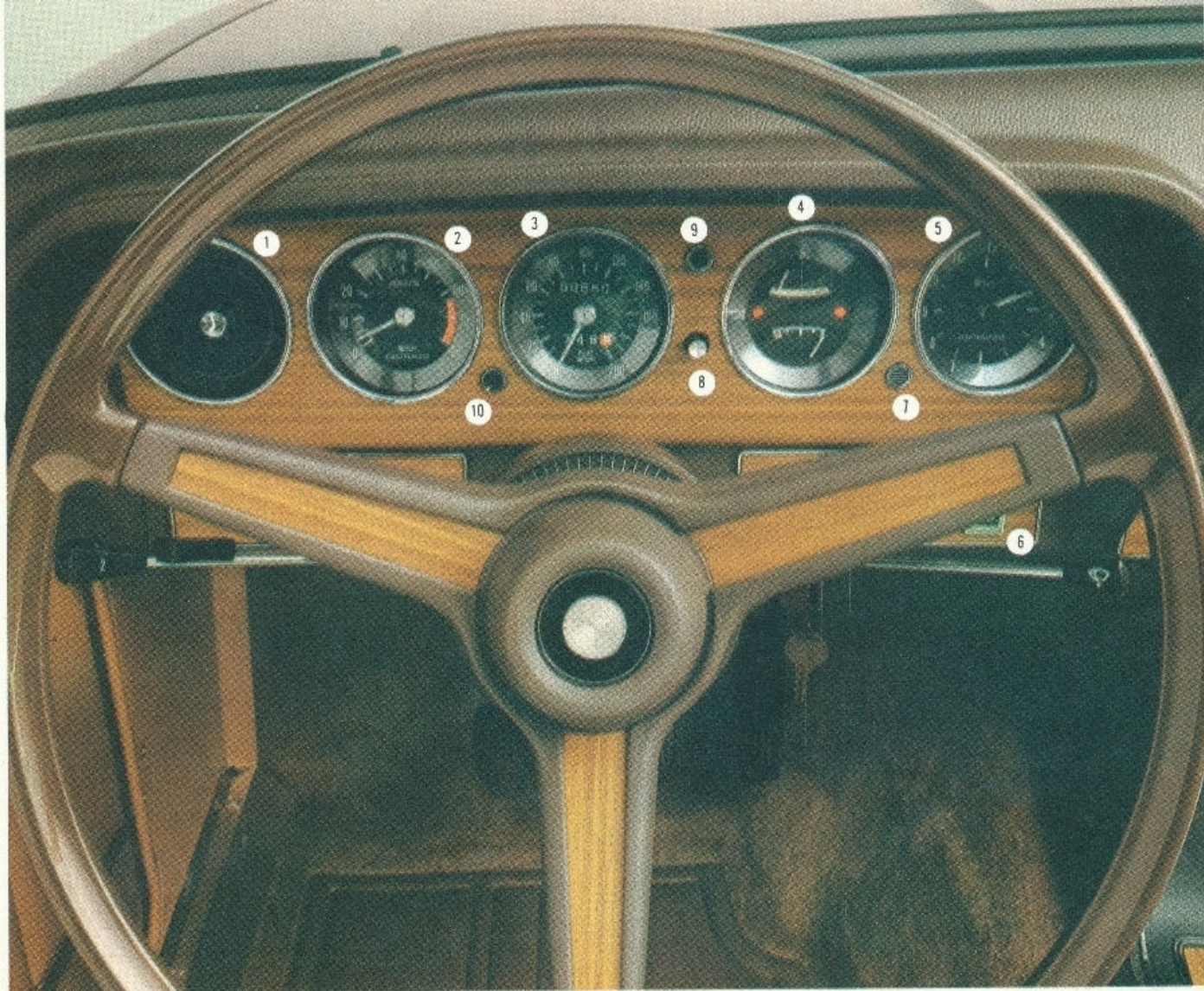
1 - Usměrnitelné větrání. - 2 - Otáčkoměr. - 3 - Ukazatel rychlosti s denním počítadlem. - 4 - Měrka benzínu se světelným signálem minimální zásoby, teploměr vody, kontrolky nabíjení a oleje. - 5 - Elektrické hodiny. - 6 - Sdružené ovládání stěrače a umývače skla. - 7 - Kontrolka silničních světlometů. - 8 - Uvedení na nulu denního počítadla. - 9 - Opakování blikáču. - 10 - Kontrolka parkovacích světel.
