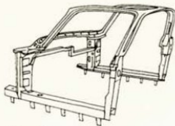
Sport Coupe framework
