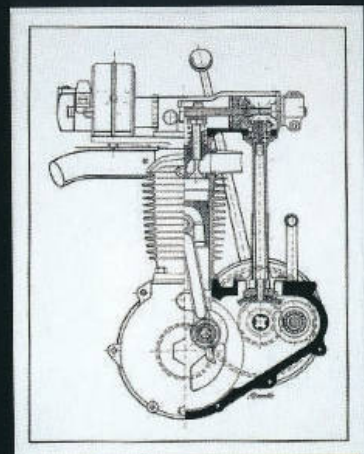
Řez motorem
